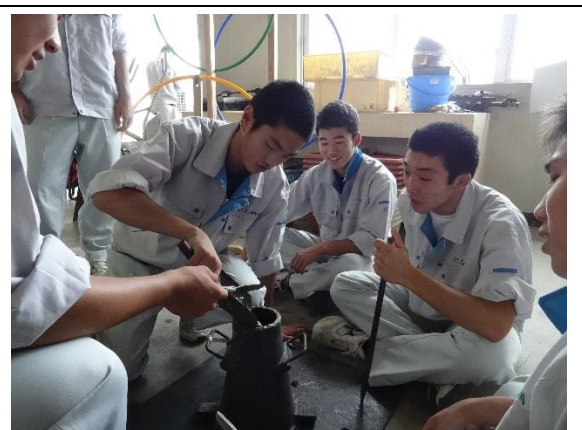
コンクリートのスランプ試験
